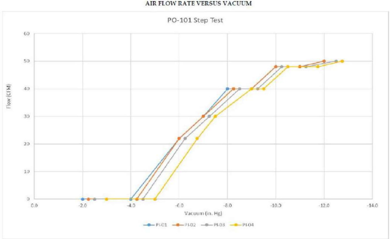
Şekil 4.7- TGE artan vakum basamağı testi örneği (Menozzi vd., bkz. Ek1)
