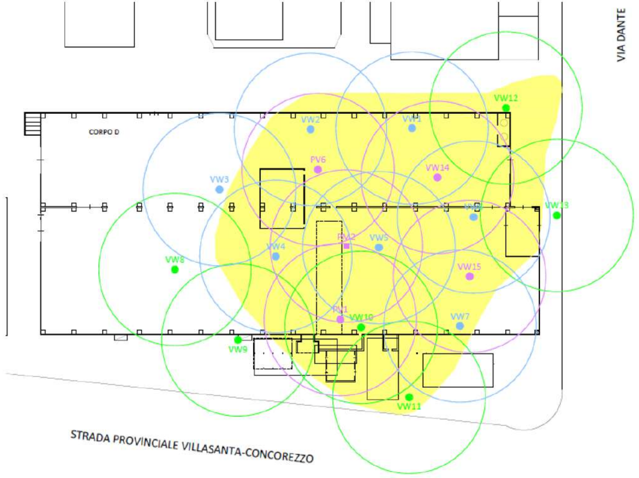
Şekil 4.1- Pilot test sonrası etki yarıçapı (Confalonieri vd., bkz. Ek1)
