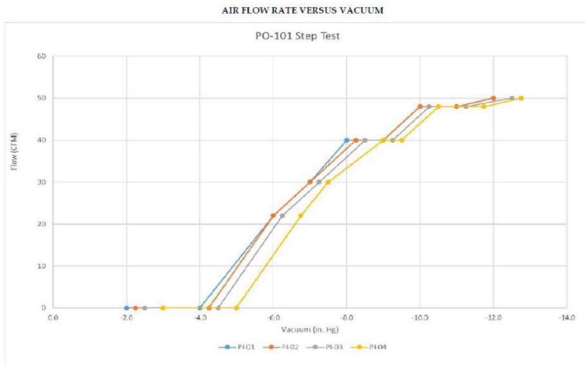
Obrázok 4.7 – Príklad krokového podtlakového testu SVE (Menozzi et al., viď Príloha 1)
