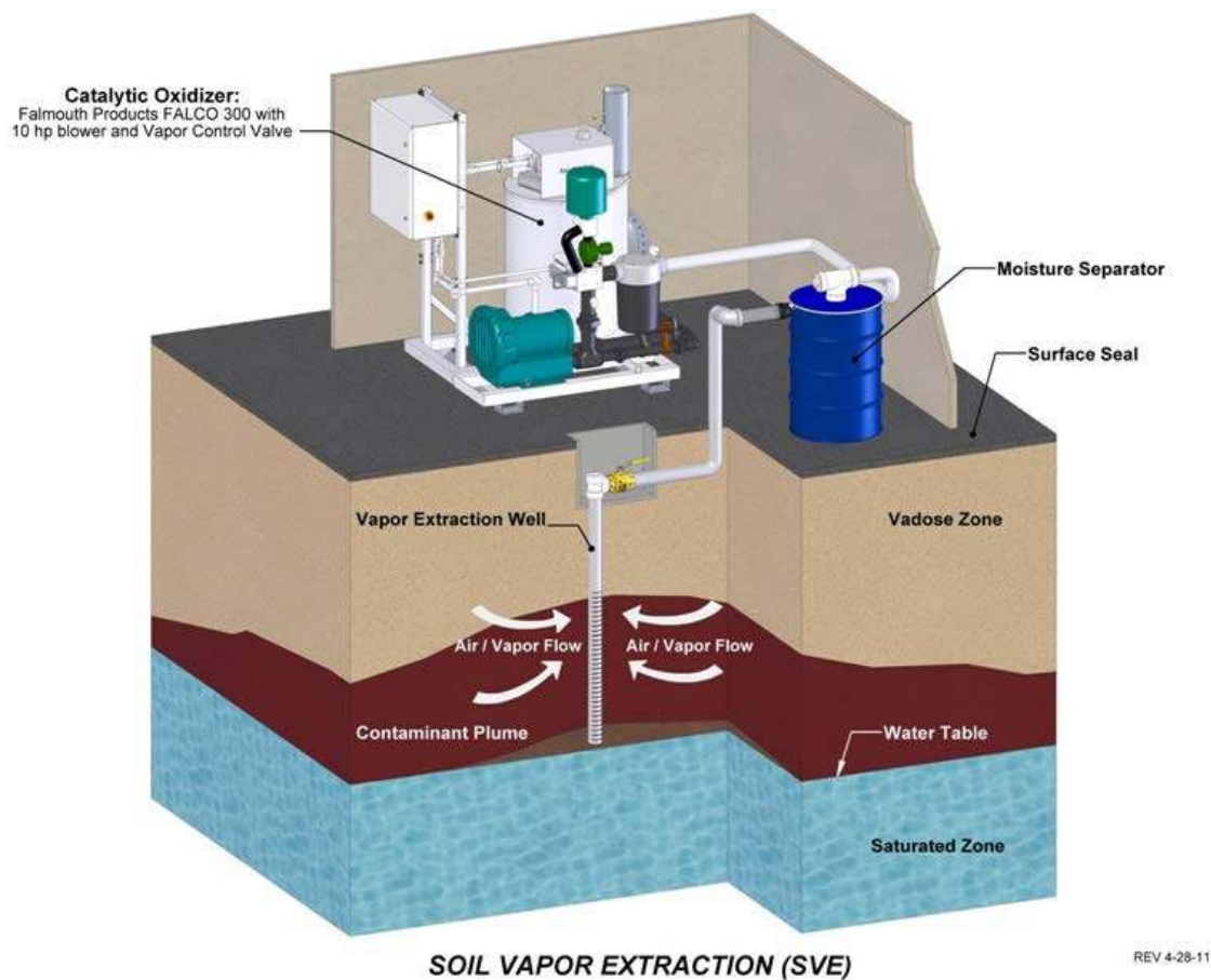
Slika 1.1- shema delovanja SVE.
