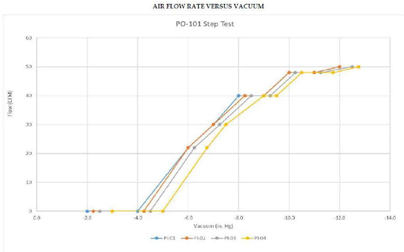
Slika 4.7- Primer preizkusa stopnje povečanja vakuuma SVE (Menozi et al., see Annex1)
