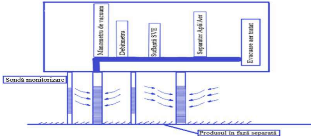
Figura 2.1- Componentele instalației SVE
