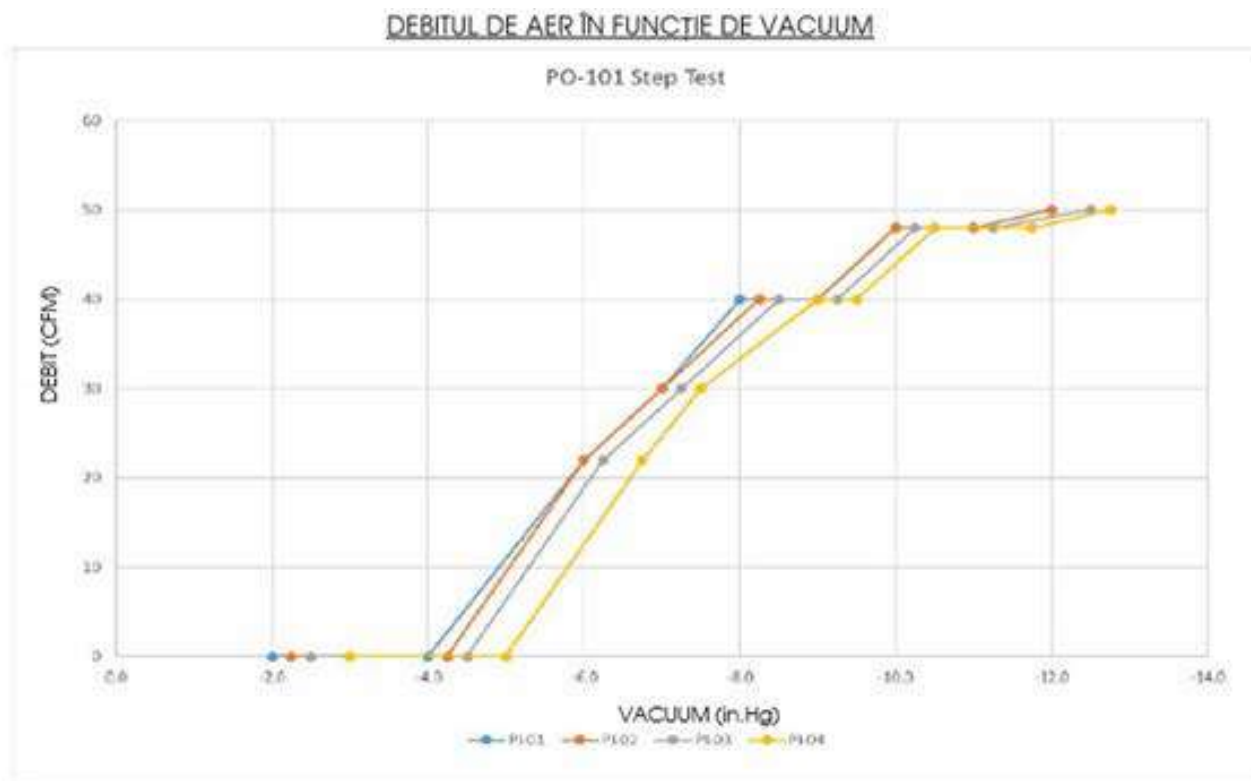
Figure 4.7- Exemplu de test de creștere a vidului în trepte SVE (Menozi et al., vezi Anexa 1)
