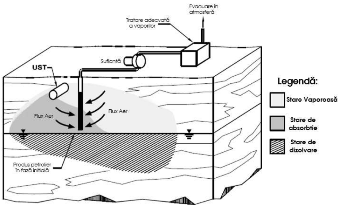
Figura 4.1- Schema cu o sursă de aer
