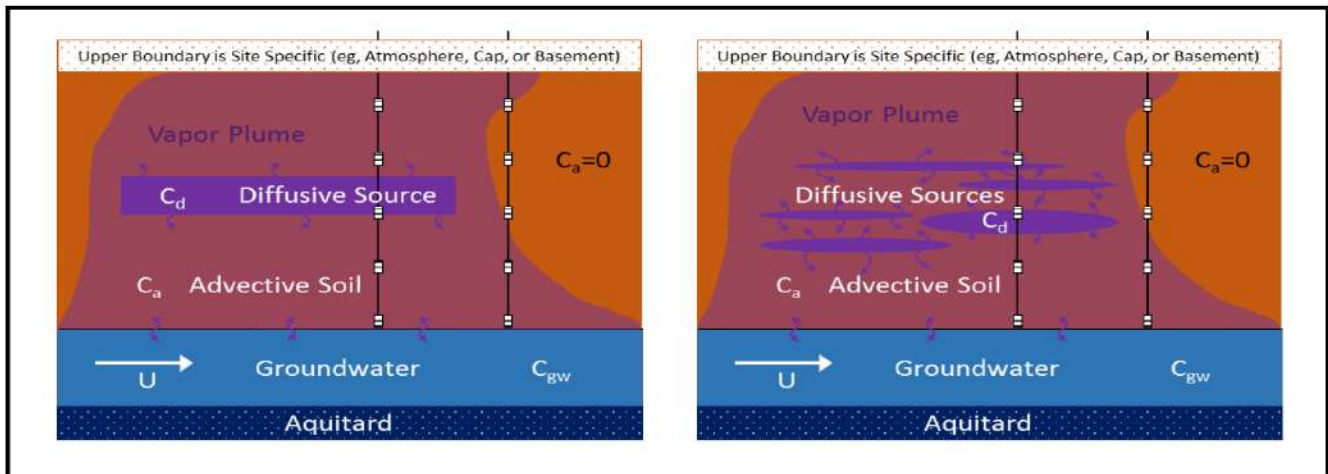
Figura 4.3- Cenários conceituais para a transferência de massa limitada por difusão e pontos típicos de monitorização de gás do solo
