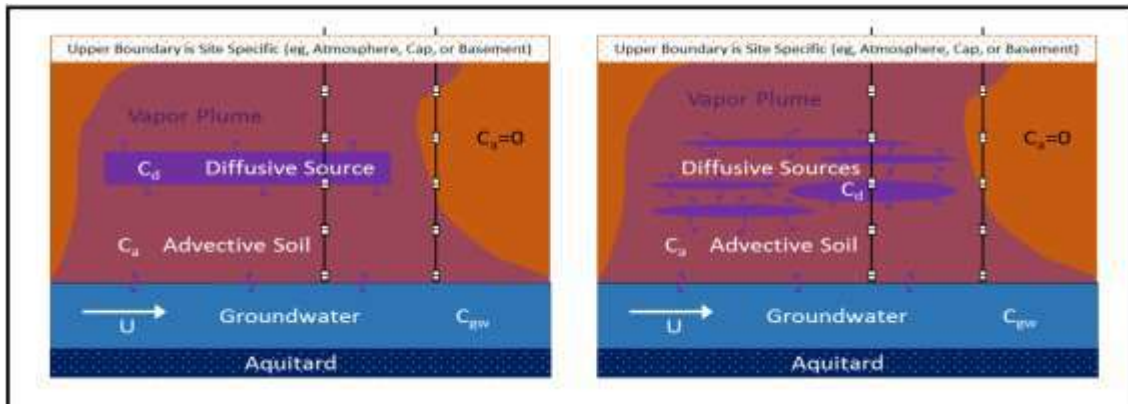
Figura 4.3- Scenari concettualizzati per il trasferimento di massa limitato alla diffusione e punti tipici di monitoraggio di soil gas
