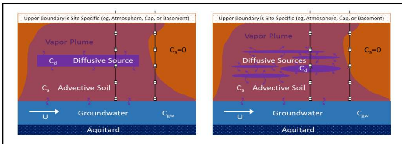
Figura 4.3 --Escenarios conceptualizados para transferencia de materia limitada por difusión y puntos típicos de control de gas en el suelo
