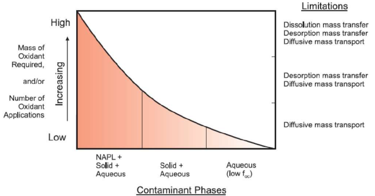
Şekil 3.2- Kirlenici fazların, kütle aktarımının ve kütle aktarım sınırlamalarının oksidanın kütlesi ve/veya ISCO için gereken oksidan uygulamalarının sayısı üzerindeki etkisi
