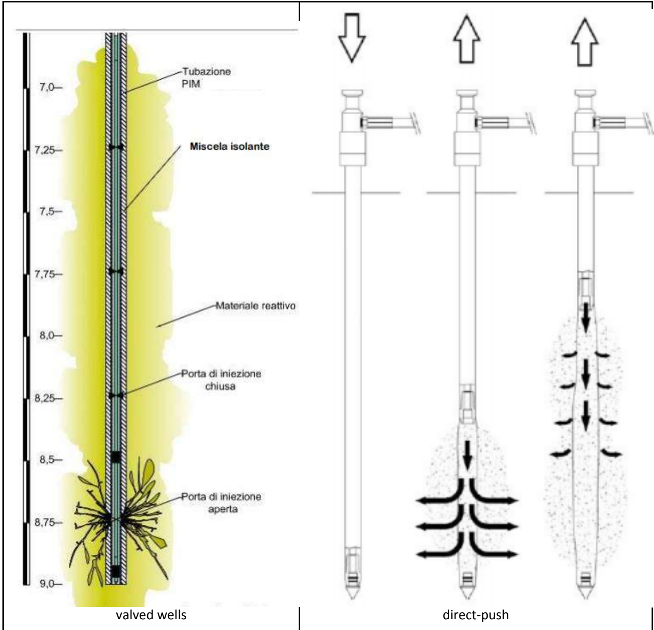
Şekil 4.2 – Valfli kuyular ve Direct-push enjeksiyon teknolojileri ( https://www.carsico.it/servizi/ )
