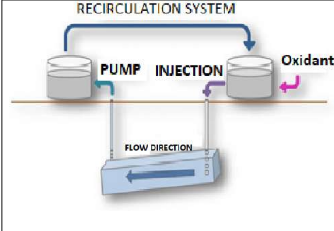
Şekil 2.2- Şema devridaim sistemi
