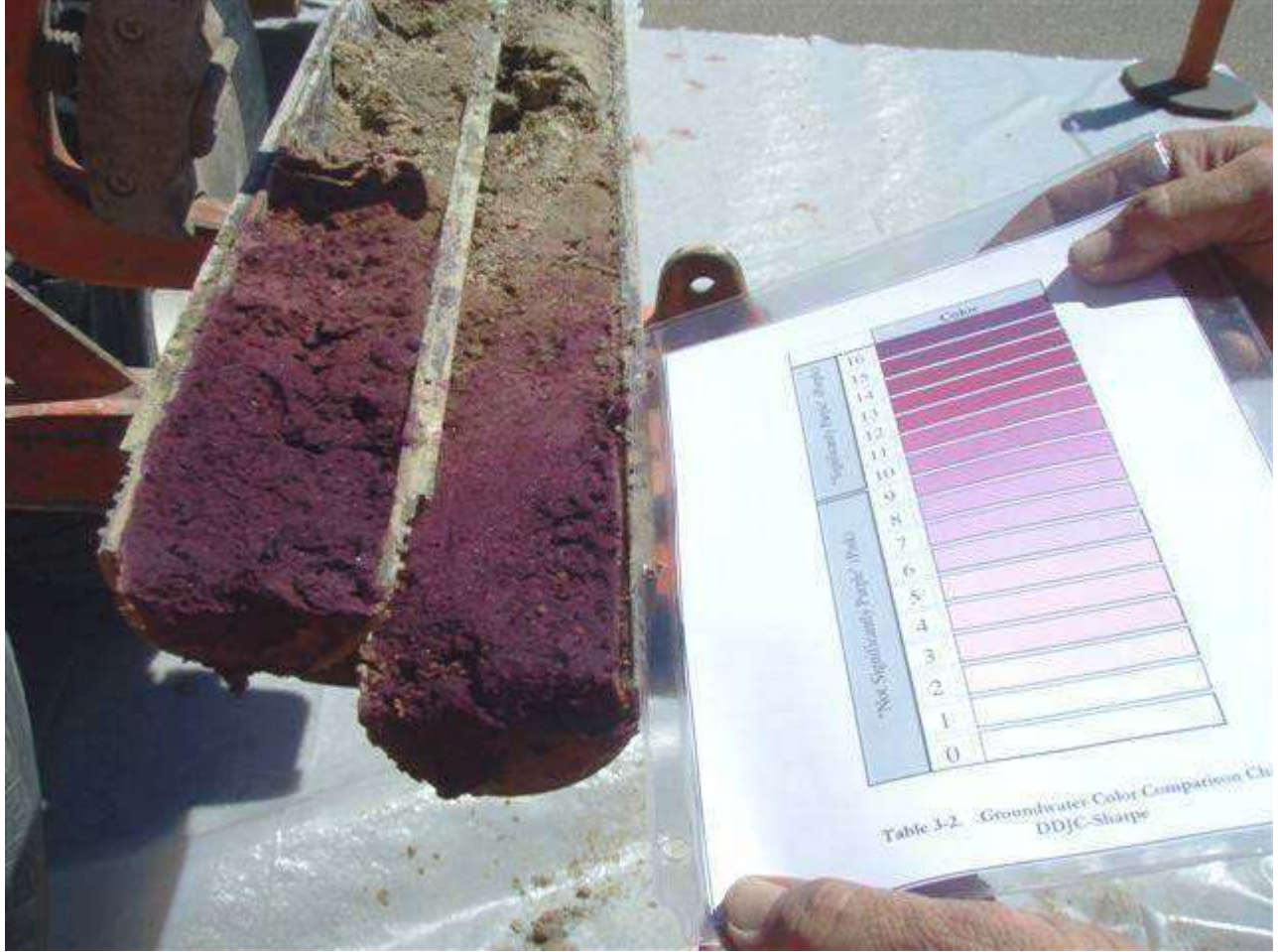
Şekil 2.8- Potasyum permanganat oksidan bulamacının kırılma-yerleşmesinden 90 gün sonra silt toprak çekirdeklerinde oksidan difüzyon profili örneği (URS'nin izniyle, Bures arşivi)
