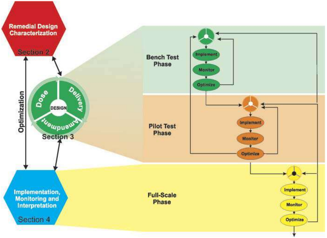
Şekil 1.2- ITRC'den şema ( https://ois-isrp-1.itrcweb.org/ )
