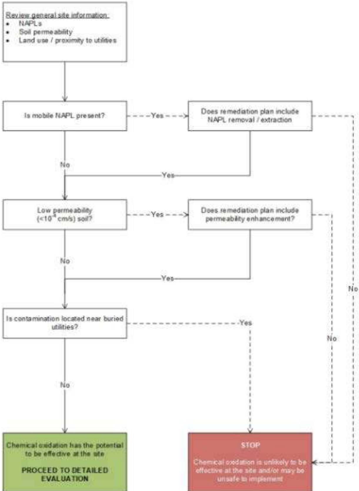
Şekil 3.1- US EPA'dan (2004) ISCO'nun potansiyel etkinliği için ilk tarama
