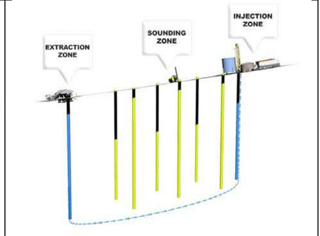
Şekil 2.3- 2D Şema devridaim sistemi
