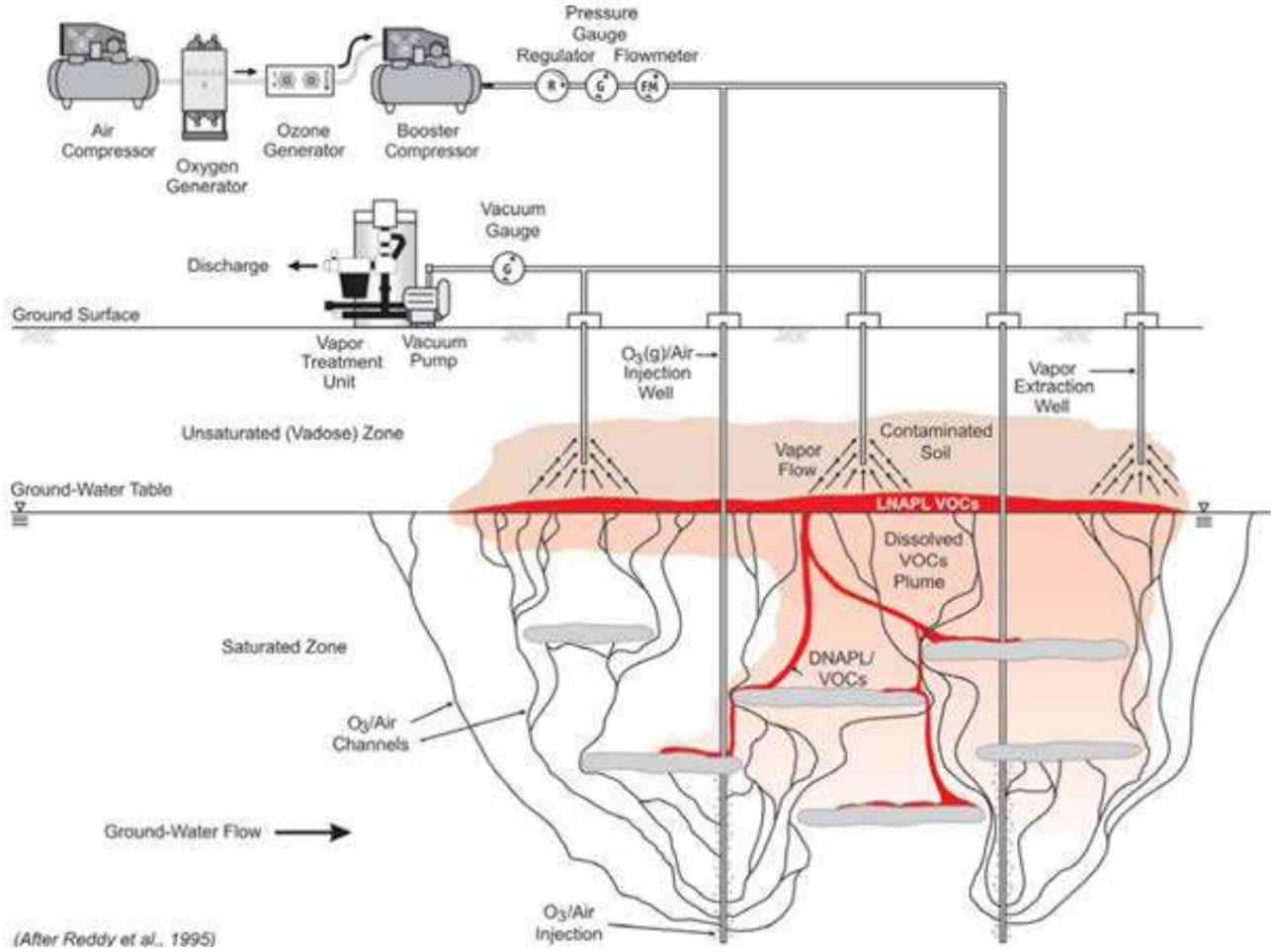
Şekil 2.9- Uçucu emisyonları ve O 3 'ü yakalamak için toprak vakum ekstraksiyonu ile doymuş bölgede yerinde ozonlamanın genel kavramsal modeli.
