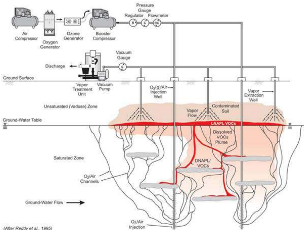
Slika 2.9- Splošni konceptualni model ozoniranja in situ v nasičenem območju z vakuumsko ekstrakcijo tal za zajemanje hlapnih emisij in O 3 .
