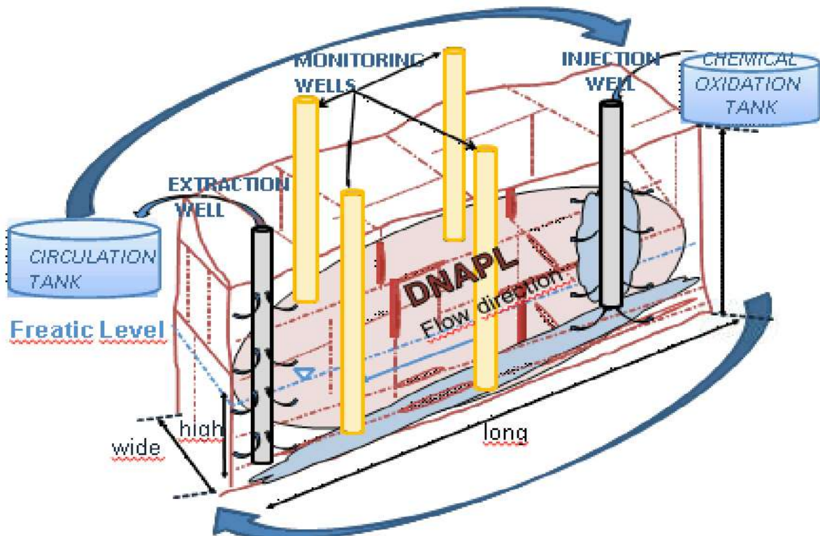
Slika 2.4- 3D Shema recirkulacijskega sistema
