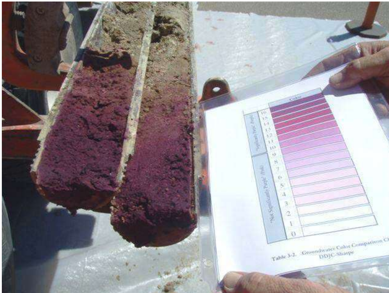
Slika 2.8- Primer profiliranja difuzije oksidantov v jedrih muljnih tal 90 dni po vgradnji oksidacijske brozge kalijevega permanganata (fotografija z dovoljenjem URS, arhiv Bures)
