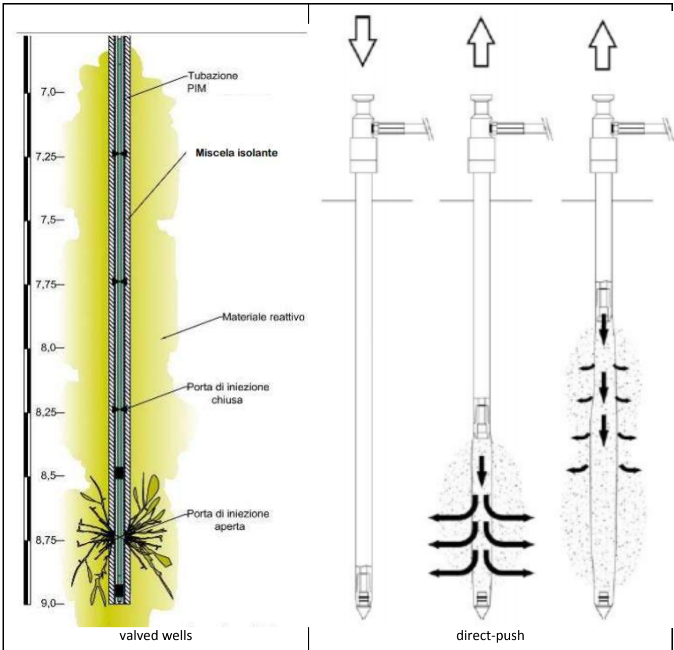
Preglednica 4.2 – Ventilne vrtine in tehnologije neposrednega vbrizgavanja ( https://www.carsico.it/servizi/ )
