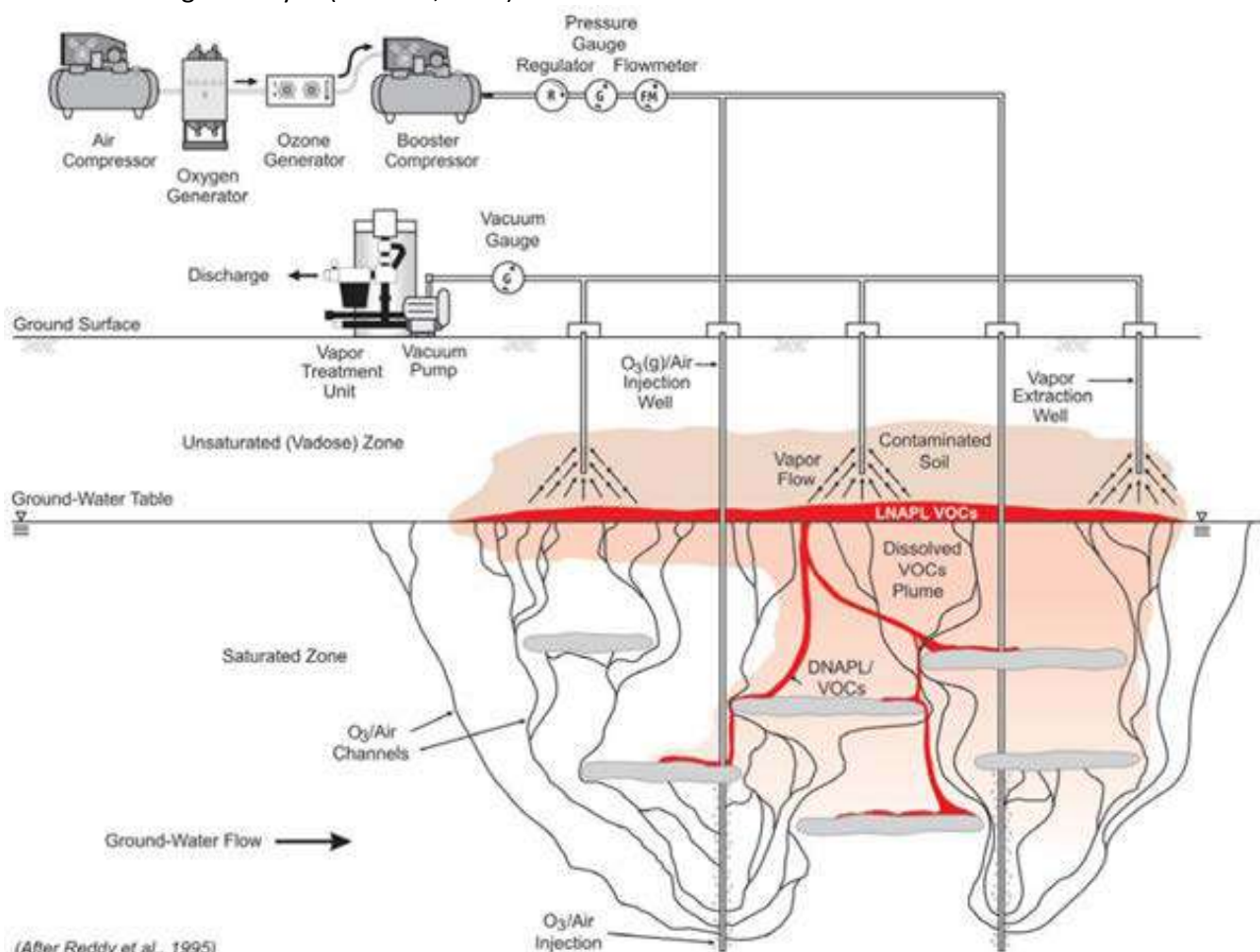
Rysunek 2.9- Ogólny model koncepcyjny ozonowania in situ w strefie saturacji z odciąganiem próżniowym z gruntu w celu wychwytywania emisji LZO i O 3
