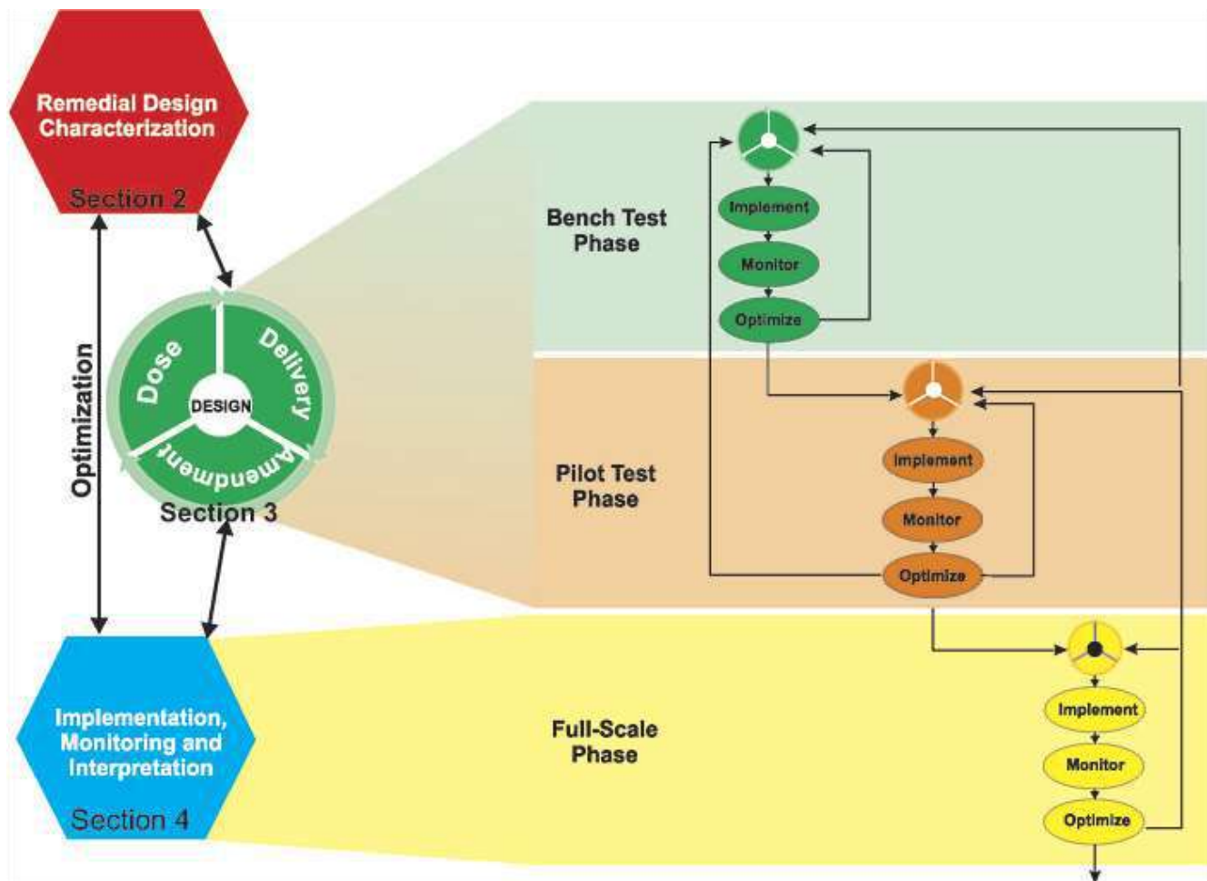
Figura 1.2- Schema del processo di bonifica (Fonte: 'ITRC - https://ois-isrp-1.itrcweb.org/ )
