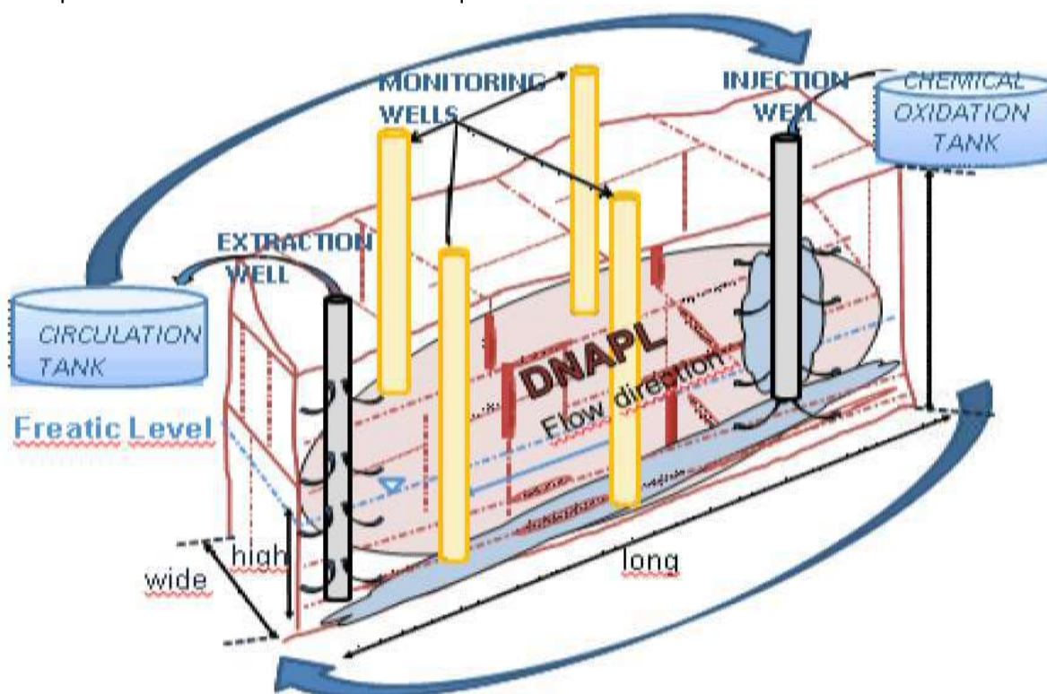
Figura 2.4- 3D Schema del sistema di ricircolo
