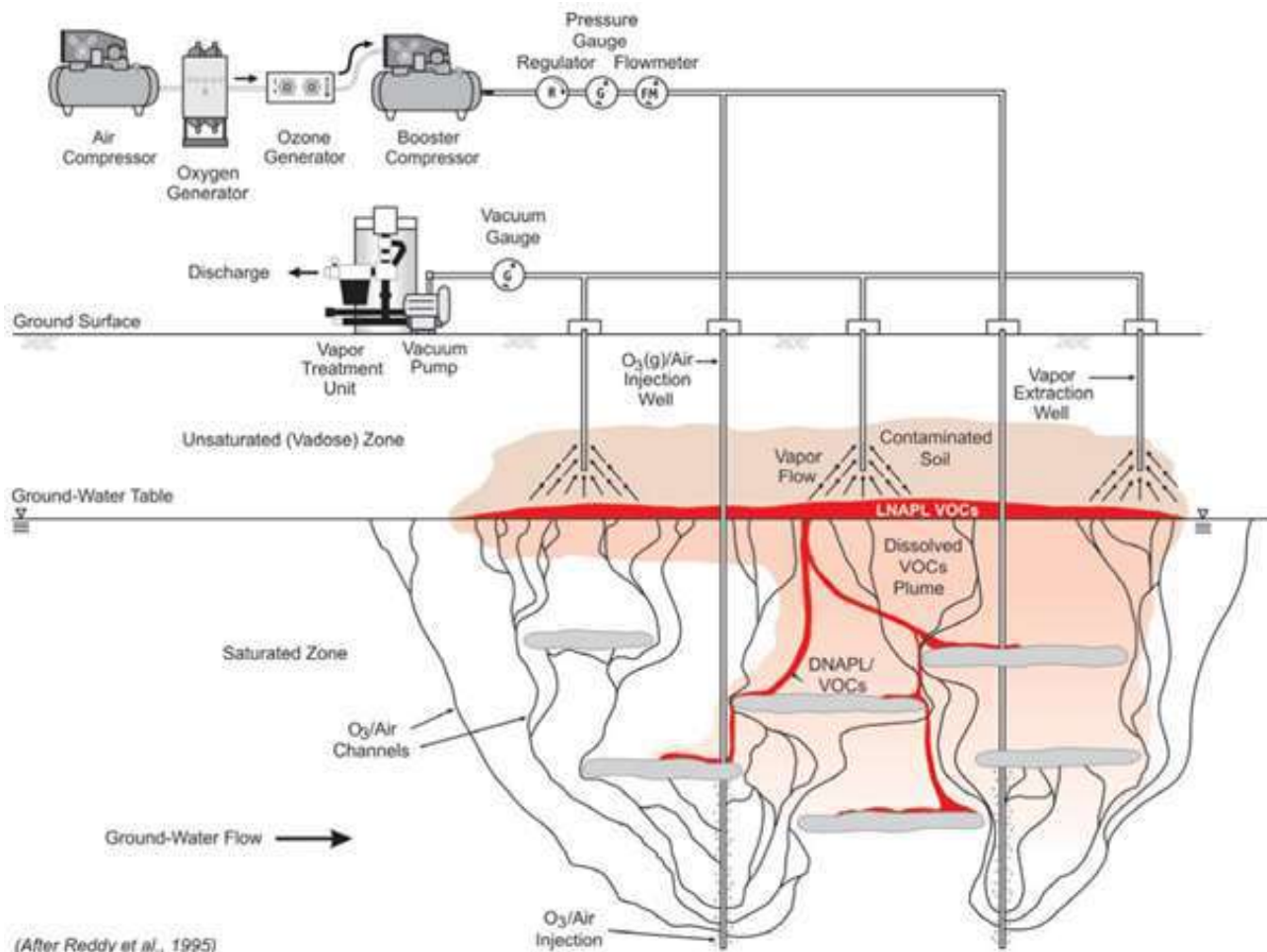
Figura 2.9- Modello concettuale generico della tecnica di iniezione di ozono nella zona satura con estrazione di vapori.
