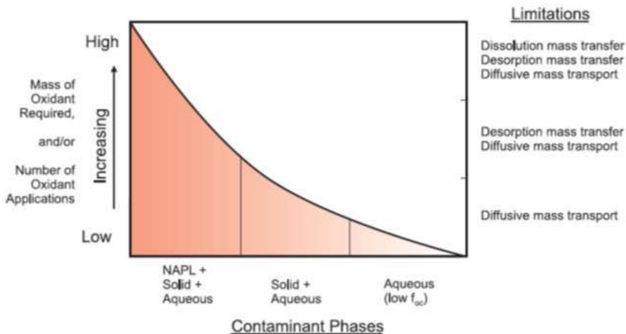
Figura 3.2- Impatto delle fasi contaminanti, trasferimento di massa e limitazioni del trasporto di massa sulla massa dell'ossidante e/o sul numero di applicazioni ossidanti necessarie per ISCO
