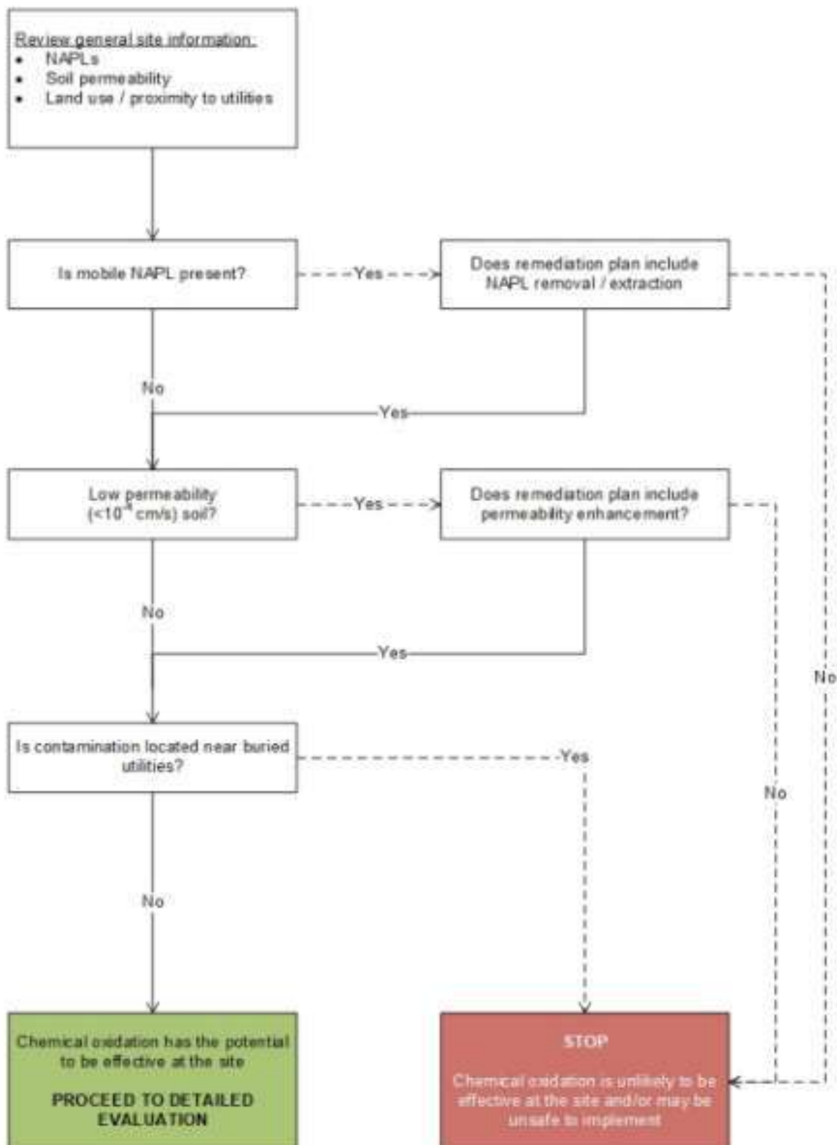
Figura 3.1- Screening iniziale per la potenziale efficacia dell'ISCO, da US EPA (2004)
