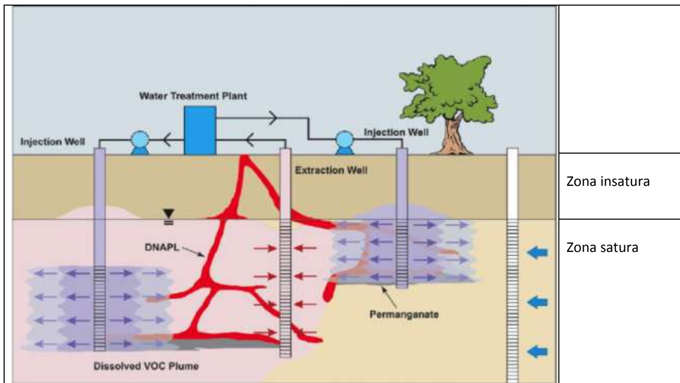
Figura 2.1- Schema dell'applicazione della tecnologia ISCO
