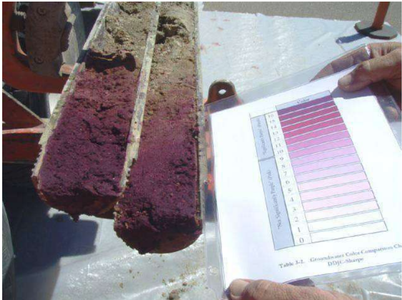
Figura 2.8- Esempio di profilo di diffusione dell'ossidante in carote di terreno di limo 90 giorni dopo l'iniezione di slurry di permanganato di potassio (foto per gentile concessione di URS, archivio Bures)
