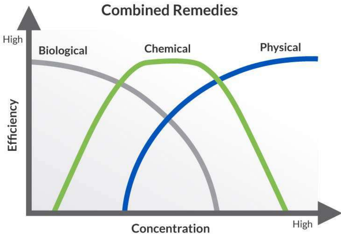
Εικόνα 1.4- Σχήμα από την Ολοκληρωμένη Θεραπεία/Επισκόπηση των Συνεργατικών Τεχνικών Αποκατάστασης (©Regenesis 2016)
