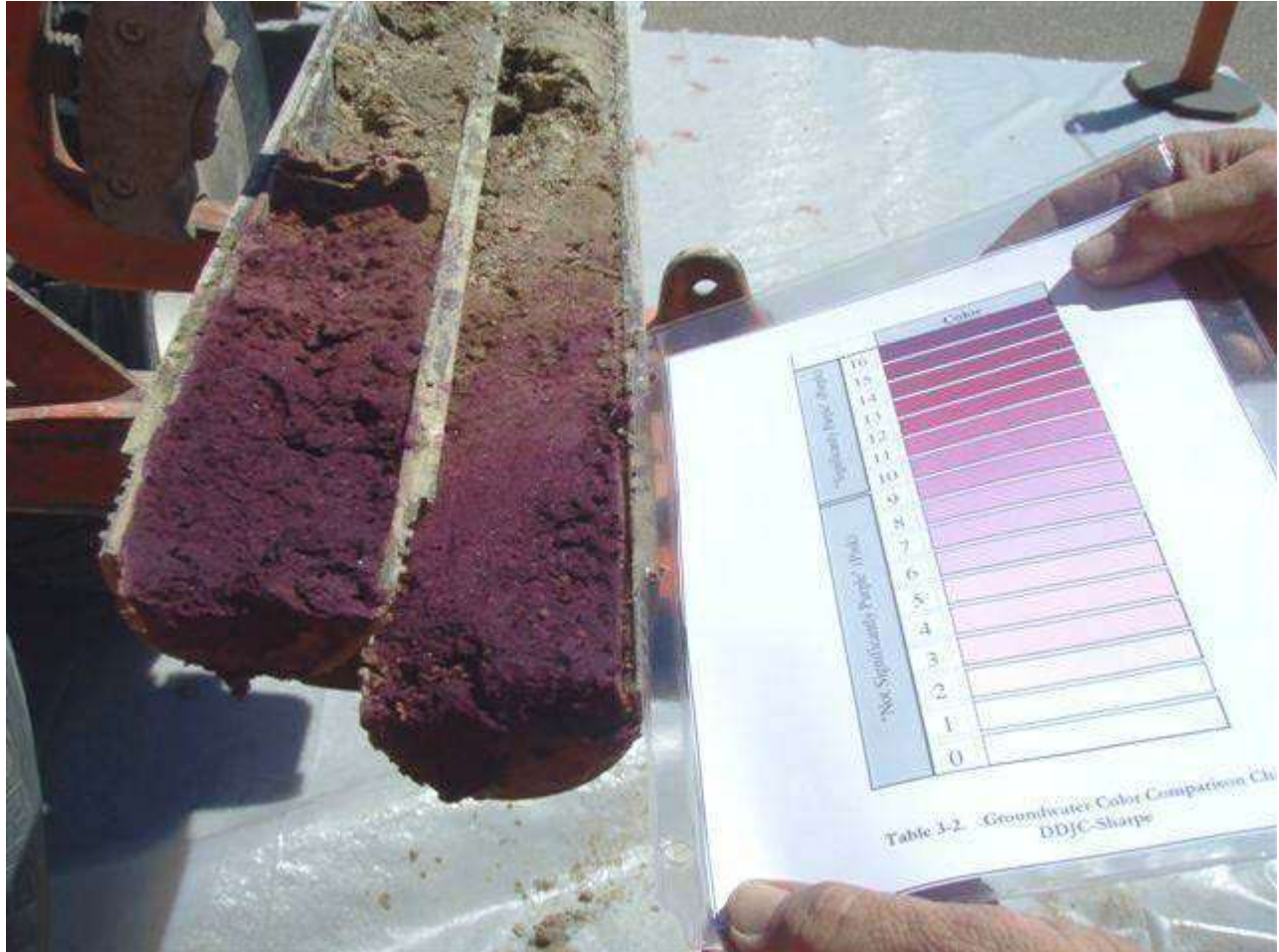
Εικόνα 2.8- Παράδειγμα προφίλ διάχυσης οξειδωτικού μέσου σε πυρήνες λυώδους εδάφους 90 ημέρες μετά τη θραύση-τοποθέτηση οξειδωτικού αιωρήματος υπερμαγγανικού καλίου (φωτογραφία με την ευγενική χορηγία της URS, αρχείο Bures)
